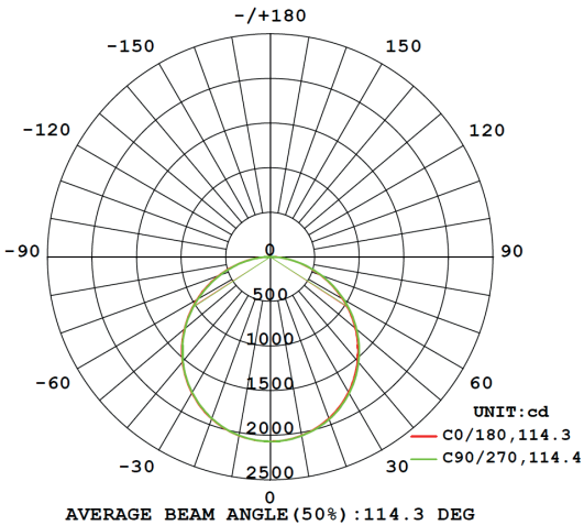
LVK Polar
