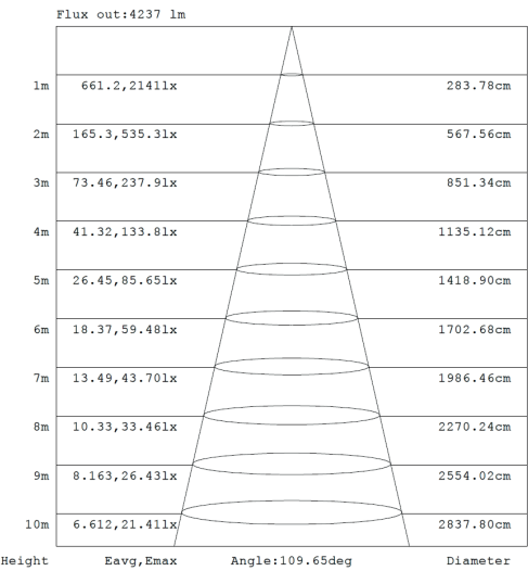
LVK Kegel
