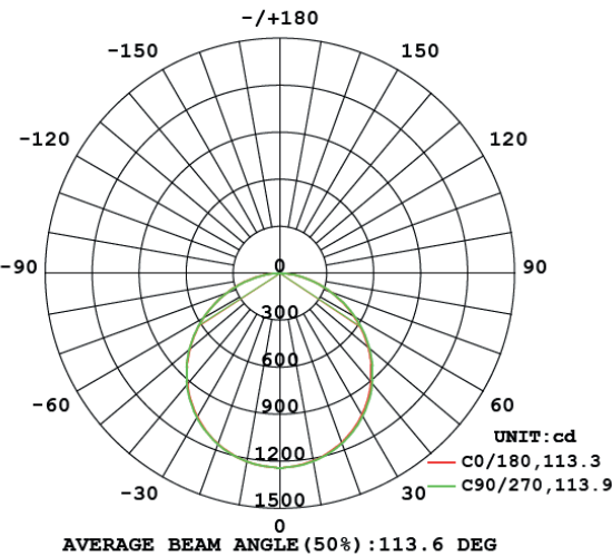
LVK Polar
